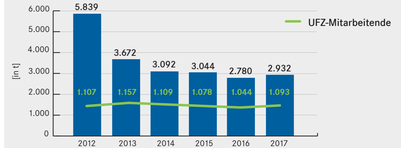
Entwicklung der CO 2 -Emissionen [in t] am UFZ
